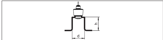
Obr. 11: Montáž do vstupního hrdla při odlišných rozměrech nátrubku
