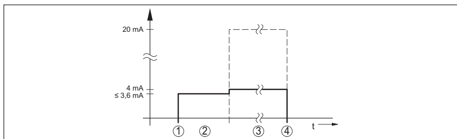
Obr. 24: Doba rozběhu a výstup naměřených hodnot
