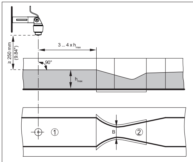
Obr. 16: Měření průtoku pomocí Khafagi-venturiho žlabu: h_{max} = max. naplnění žlabu; B = velké zúžení žlabu
