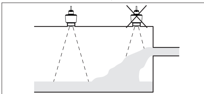
Obr. 9: Montáž radarového hladinoměru při plnění média
