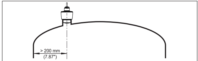
Obr. 6: Montáž radarového hladinoměru na zásobníku s kulovou střechou
