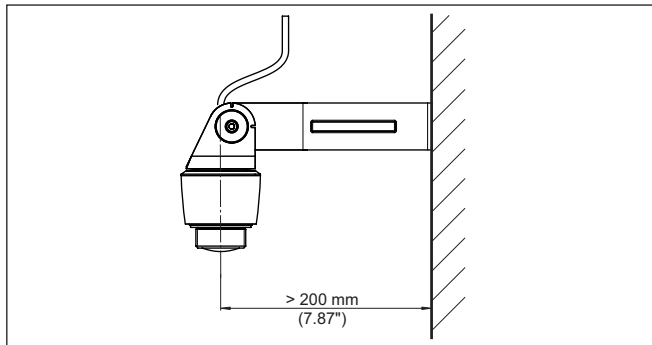
Obr. 4: Montáž pomocí montážního držáku
