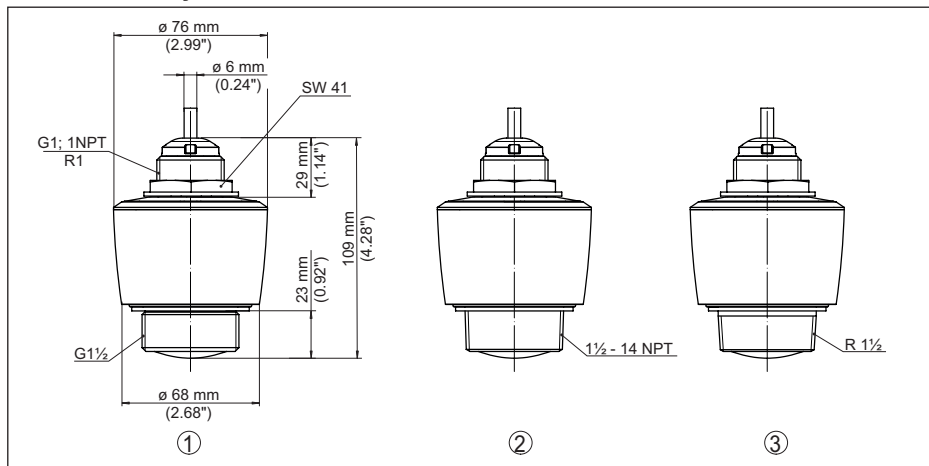
Obr. 26: Rozměry VEGAPULS C 11
