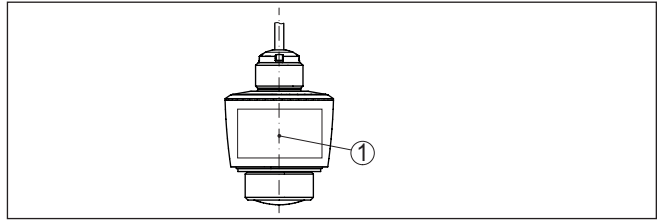
Obr. 5: Pozice polarizace
