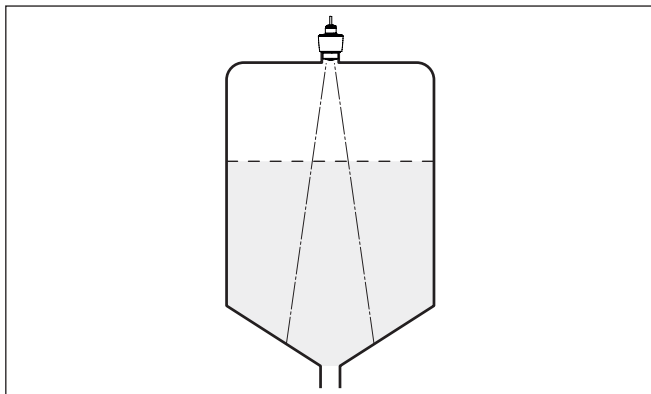
Obr. 7: Montáž radarového hladinoměru na nádrži s kuželovým dnem
