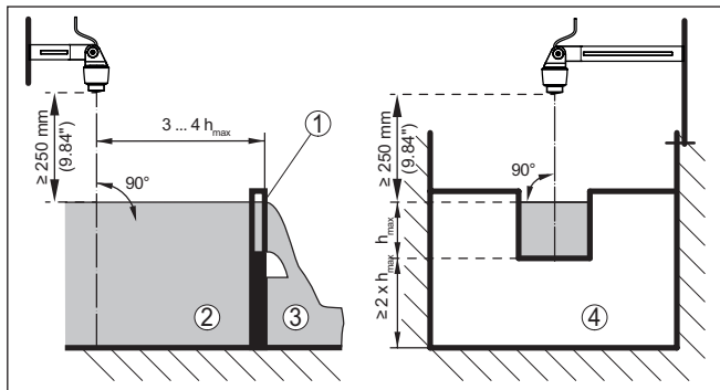
Obr. 15: Měření průtoku s pravouhlým přepadem: h_{max} = max. naplnění pravouhlého přepadu
