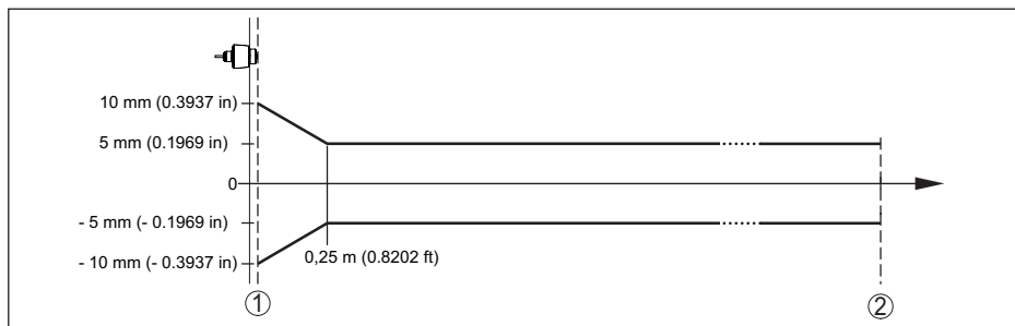
Obr. 25: Odchylka dle referenčních podmínek 10)
