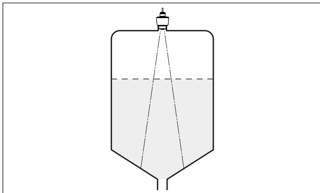
Obr. 8: Montáž radarového hladinoměru na nádrži s kuželovým dnem
