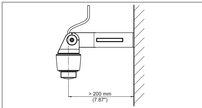
Obr. 5: Montáž pomocí montážního držáku
