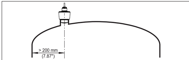
Obr. 7: Montáž radarového hladinoměru na zásobníku s kulovou střešou
