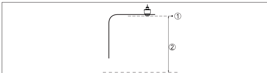
Obr. 27: Data vstupních proměnných
