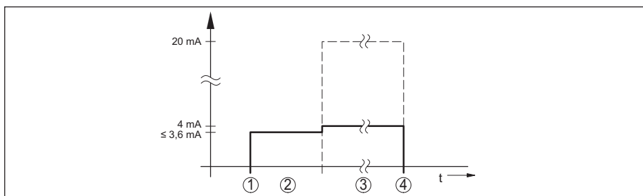
Obr. 28: Doba rozběhu a výstup naměřených hodnot
