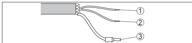
Obr. 18: Rozdělení vodičů - propojovací kabel
