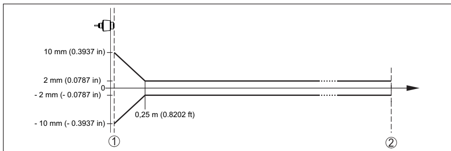
Obr. 29: Odchylka dle referenčních podmínek 11)
