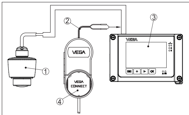
Obr. 24: Připojení PC k řídicímu přístroji VEGAMET
