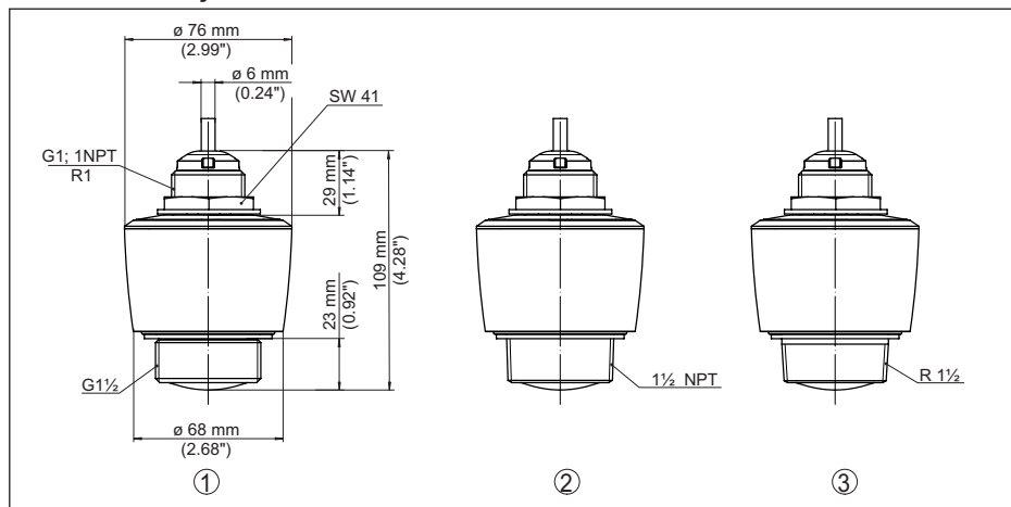
Obr. 30: Rozměry VEGAPULS C 21
