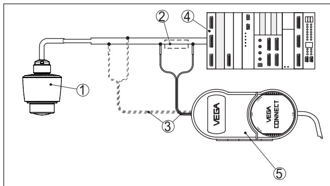
Obr. 23: Propojení s PC přes proudovou smyčku
