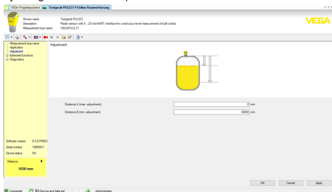
Obr. 22: Příklad jednoho náhledu DTM - Uvedení do provozu Nastavení snímače
