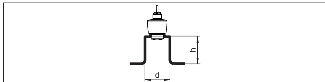
Obr. 12: Montáž do vstupního hrdla při odlišných rozměrech nátrubku
