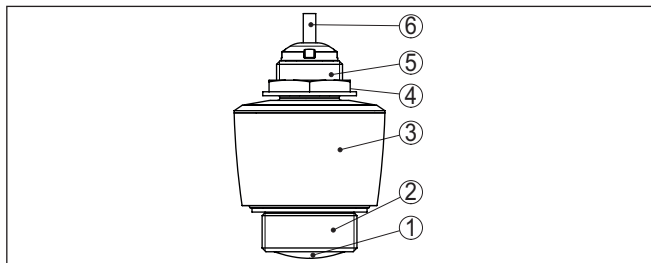
Obr. 1: Součásti přístroje VEGAPULS C 21
